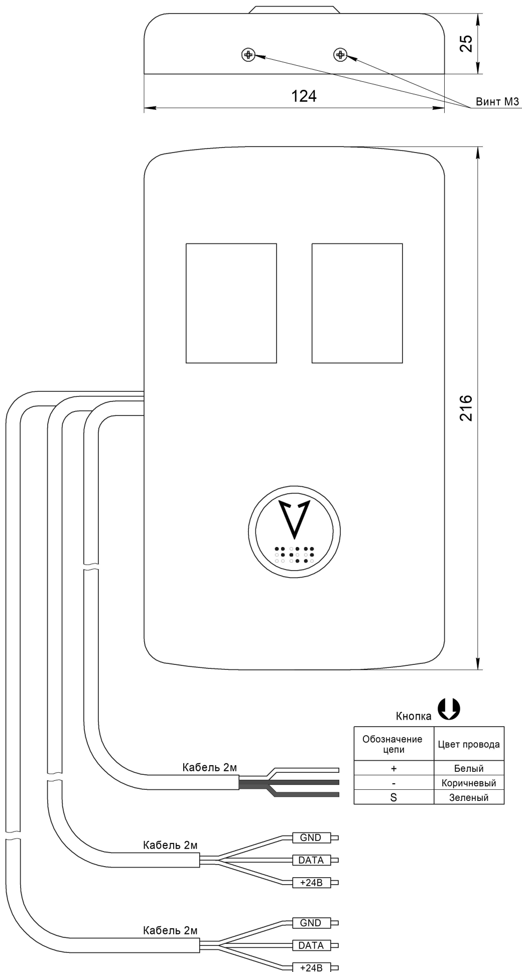
Рис.1 Внешний вид, габаритные и установочные размеры Вызывного поста ВП-1102-2074-13
